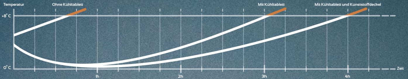
Temperaturentwicklung in zu kühlenden Lebensmitteln bei einer Umgebungstemperatur von +24 °C
